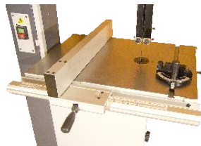
Lineal, Gehrungsanschlag Lasermarkierung
