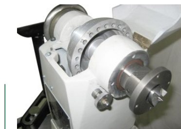
Rasterscheibe für 24 Positionen
