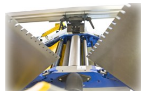
3 Messerwelle
